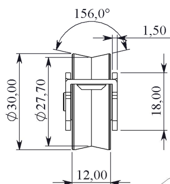
DETTAGLIO B SCALA 2 : 1
