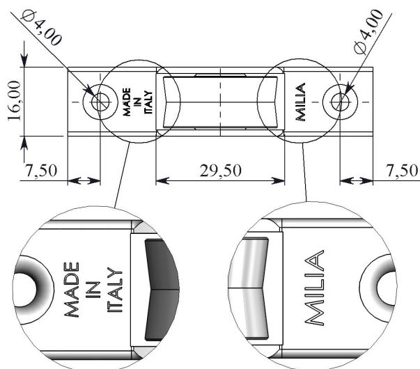
DETTAGLIO C SCALA 2 : 1
